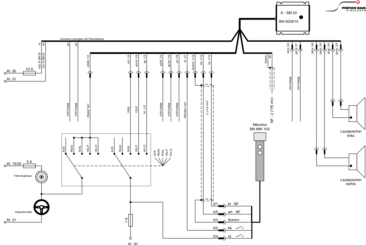
Anschlussplan mit Mikrofon - Minuseintastung -
