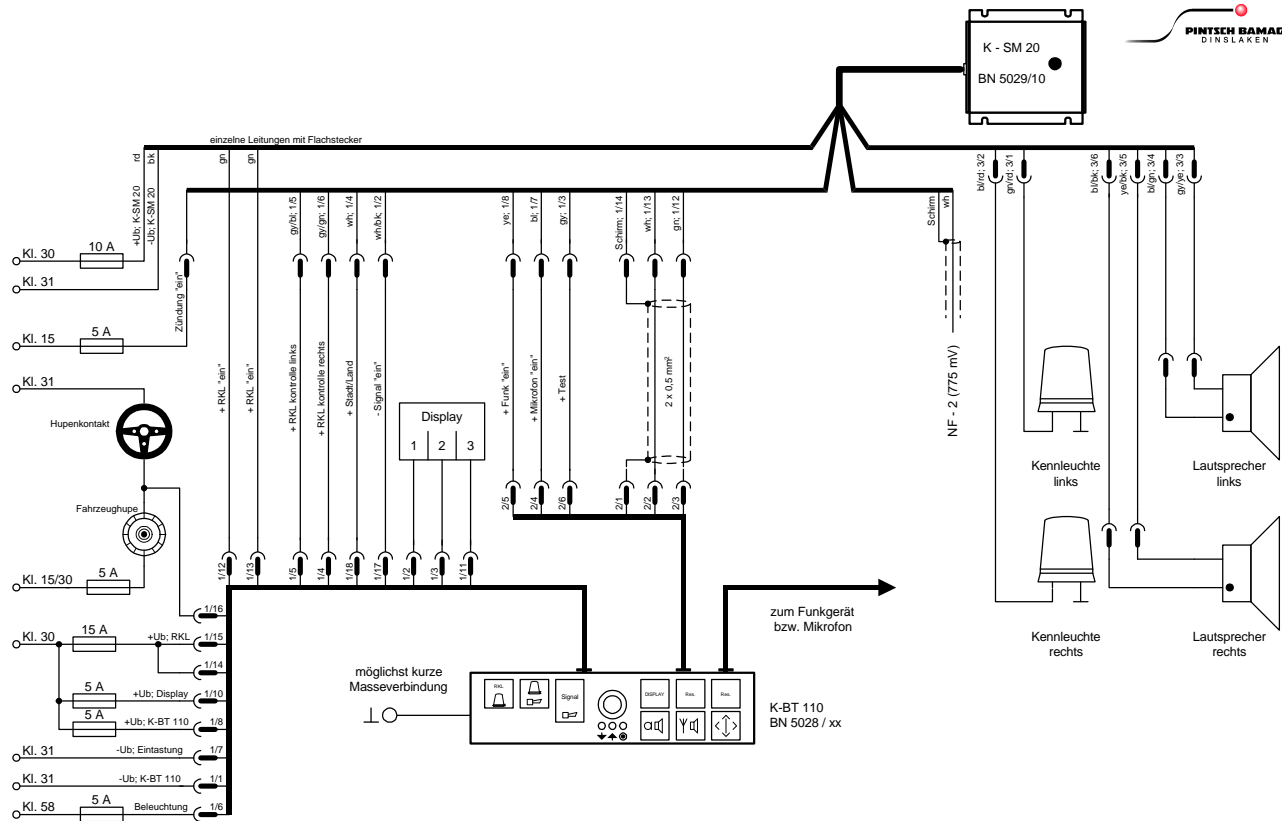
Anschlussplan mit K-BT 110 - Minuseintastung -
