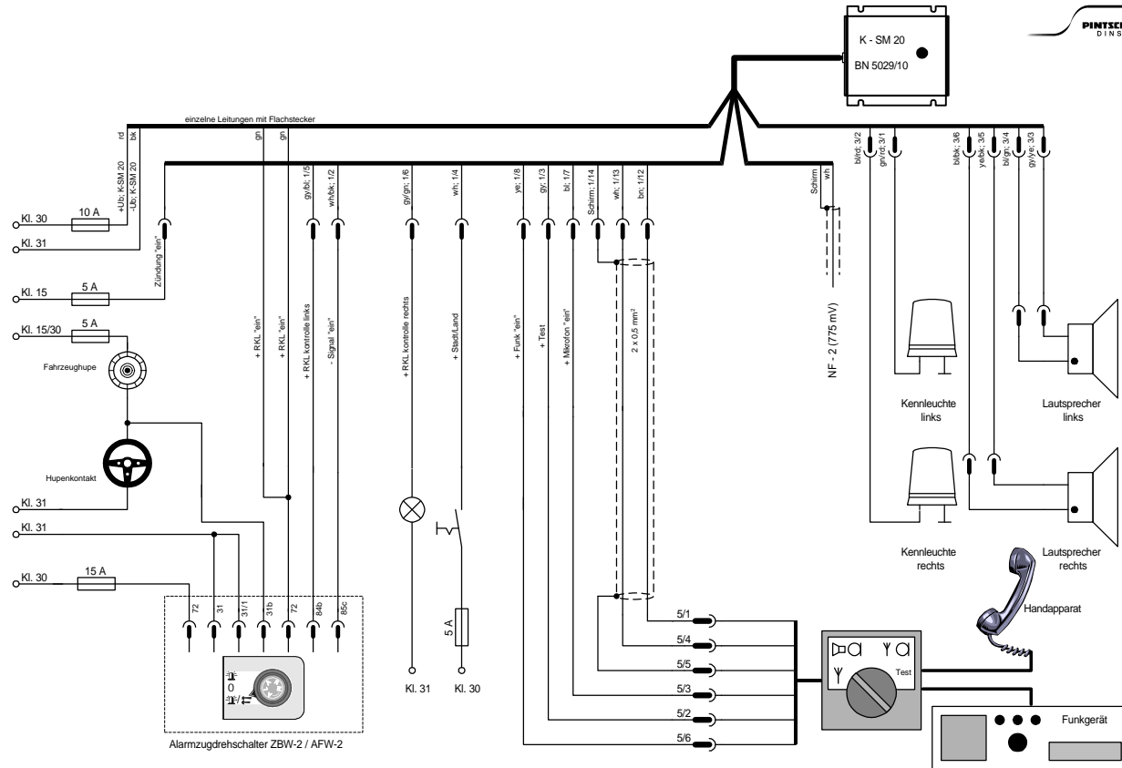
Anschlussplan mit Alarmdrehzugschalter, BT-14 - Minuseintastung -
