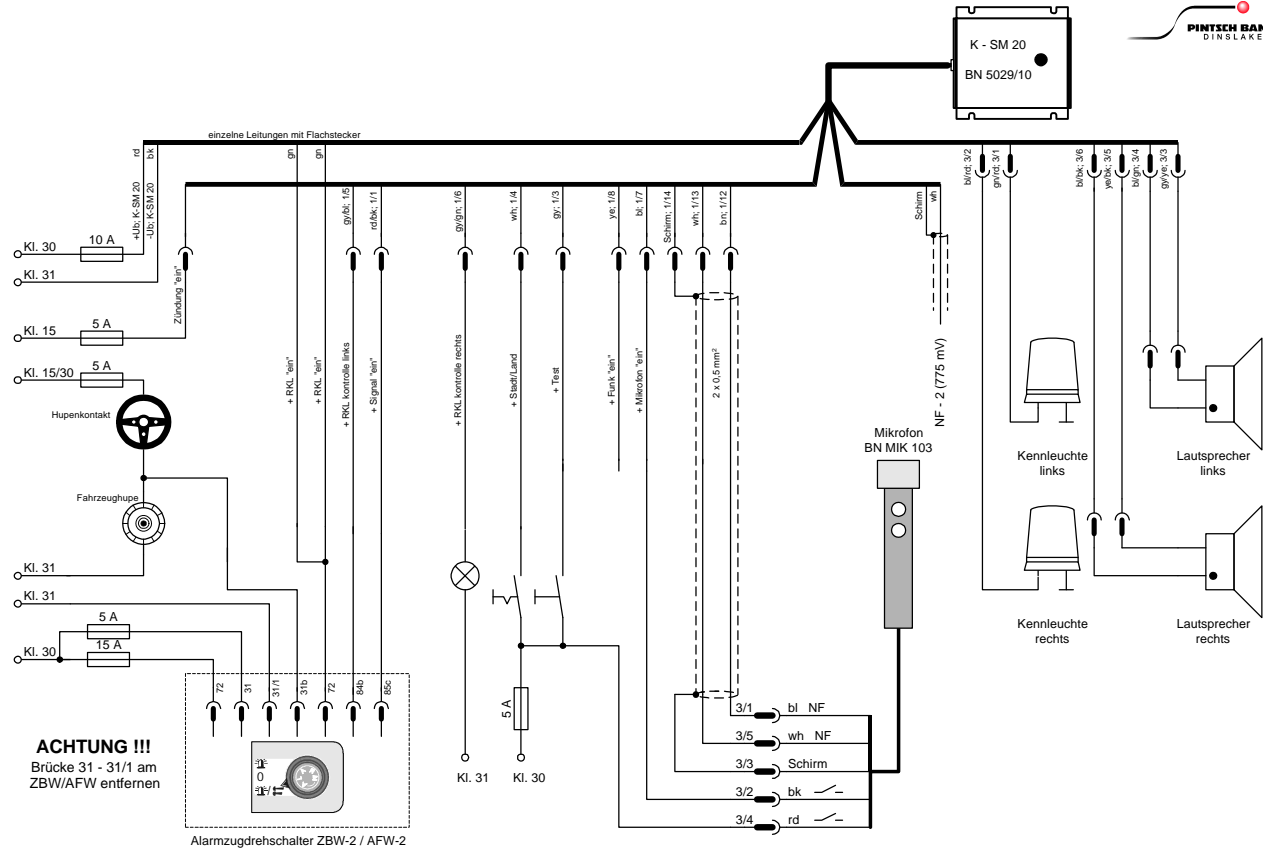
Anschlussplan mit Alarmdrehzugschalter, Mikrophon - Pluseintastung -
