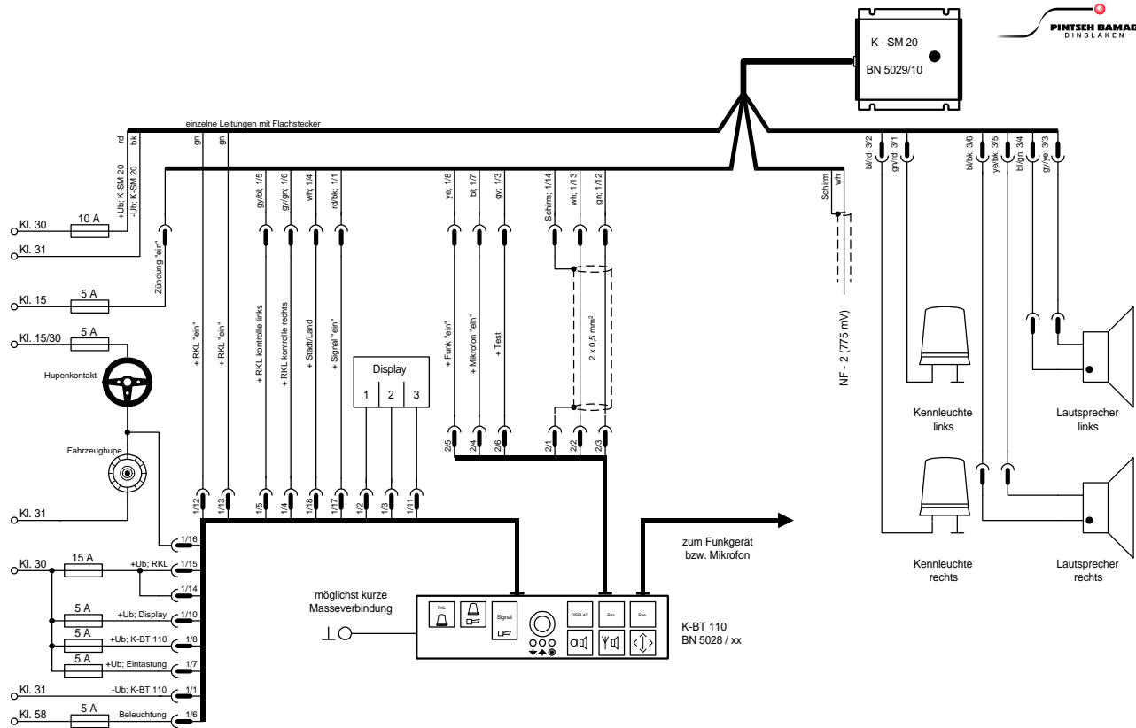
Anschlussplan mit K-BT 110 - Pluseintastung -
