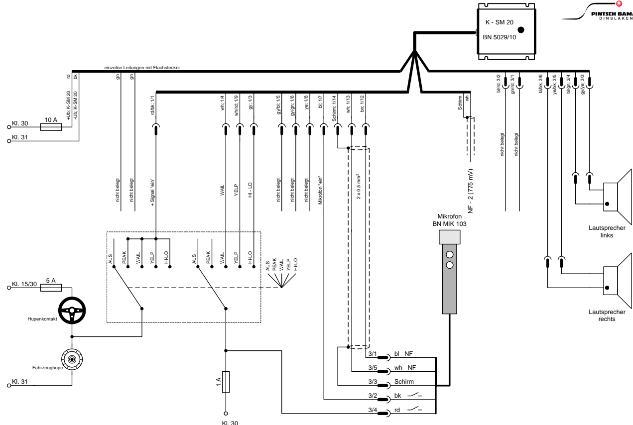
Anschlussplan mit Mikrofon - Pluseintastung -
